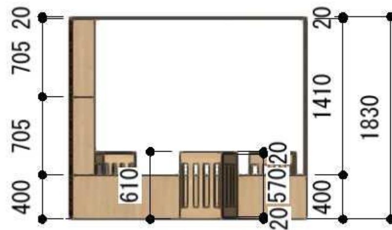
— 右側立面図 —
