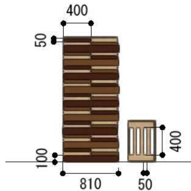
— 前側立面図 —
