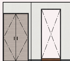
居室 北展開図
